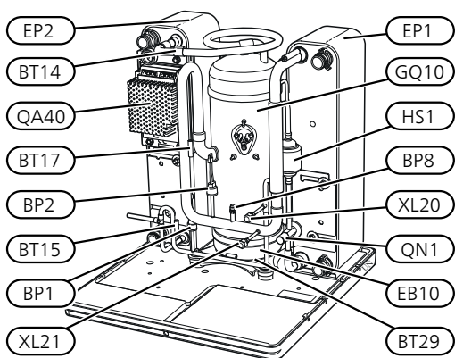
Kylmodul EP15
