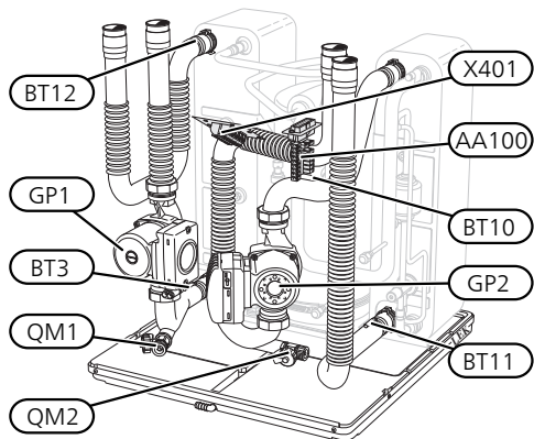
Kylmodul EP15
