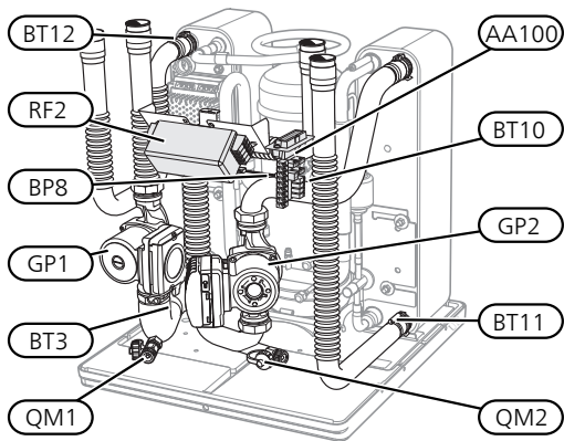
Kylmodul EP14
