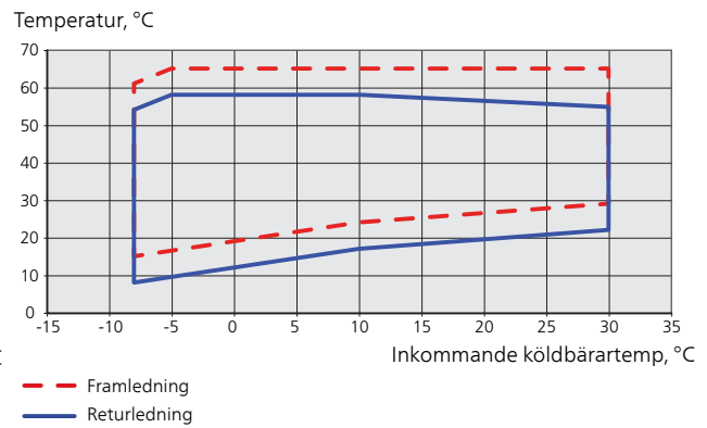
Kylmodul EP15
